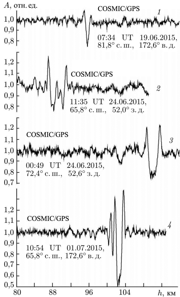
Рис. 1. Зависимости нормированной амплитуды A радиозатменного сигнала от высоты перигея луча h , полученные с помощью спутников COSMIC/GPS при зондировании четырех районов высокоширотной ионосферы Северного полушария Земли.
