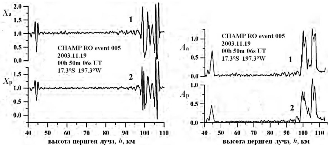
Рис. 2. Вертикальные профили X_a и X_p рефракционного ослабления, найденные из радиозатменных данных CHAMP/GPS об амплитуде (кривая 1) и эйконе (кривая 2) сигнала на несущей частоте f_1 = 1575.42 МГц. Справа показаны соответствующие амплитуды A_a и A_p аналитических сигналов (X_a - 1) и (X_p - 1) .
