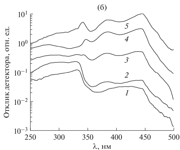
Рис. 6. Зависимость спектральной фоточувствительности МПМ-детектора Д1 (а) и Д2 (б) от напряжения смещения: а) U_{смещ} = 10 (1), 20 (2), 30 (3), 50 (4) и 60 В (5); б) U_{смещ} = 5 (1), 10 (2), 15 (3), 30 (4) и 40 В (5).
