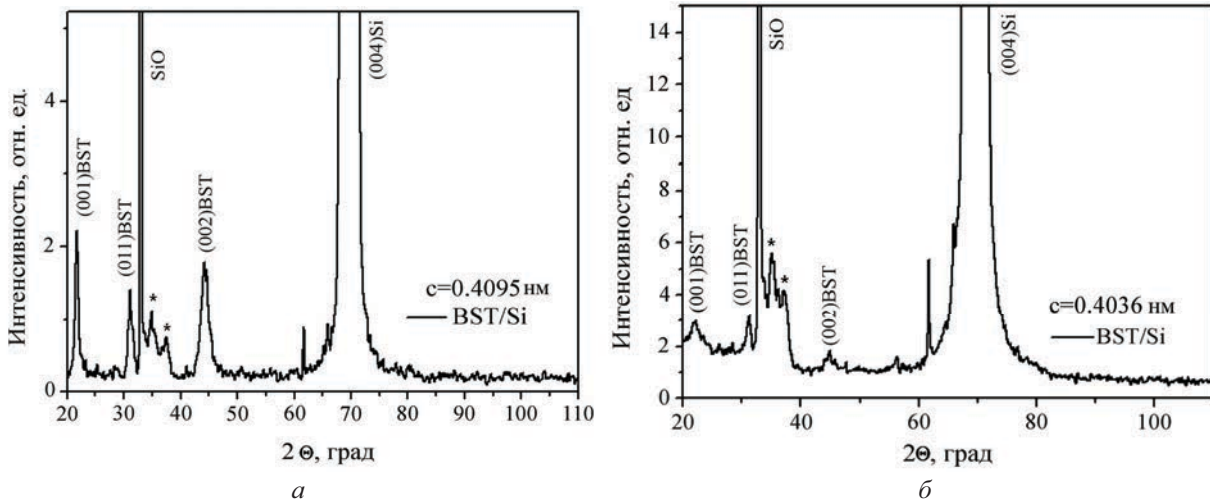
Рис. 1. Рентгенограммы плёнок \text{Ba}_{0.2}\text{Sr}_{0.8}\text{TiO}_3 на Si подложке. Толщина плёнки: a - 0.5 мкм, b - 1.0 мкм
