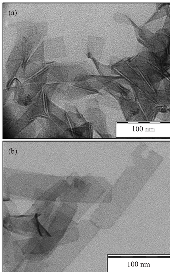
Рис. 1. ПЭМ нанопластин CdSe (а) и гетероструктур CdSe/CdS (б)
