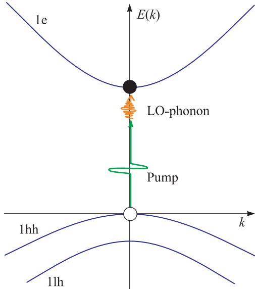
Рис. 4. (Цветной онлайн) Схема поглощения носителей с участием оптического LO-фонона в квазидвумерной системе в случае возбуждения в край области экситонного поглощения. Зеленой стрелкой указана энергия второй гармоники лазера, оранжевой стрелкой указана энергия оптического фонона
