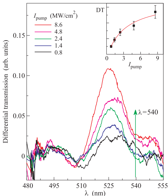
Рис. 3. (Цветной онлайн) Спектры дифференциального пропускания коллоидного раствора нанопластинок CdSe/CdS при различной интенсивности возбуждающих лазерных импульсов. Зеленой стрелкой указана длина волны второй гармоники лазера. На вставке приведена зависимость площади дифференциального пропускания от интенсивности возбуждающих импульсов
