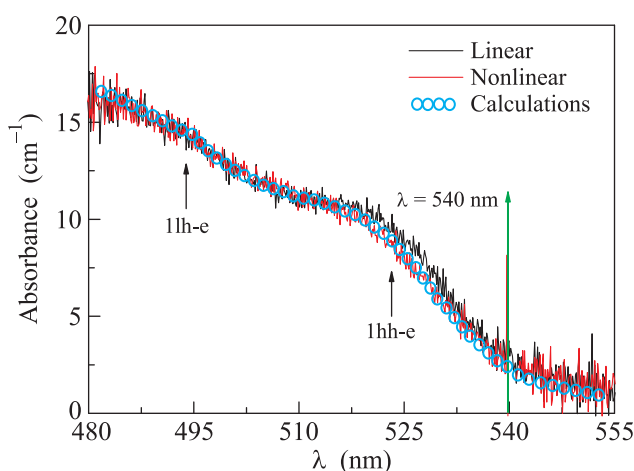
Рис. 2. (Цветной онлайн) Линейный спектр поглощения коллоидного раствора нанопластинок CdSe/CdS (черная линия) и спектр поглощения, измеренный при нерезонансной накачке лазерным излучением с интенсивностью 8.6 МВт/см 2 (красная линия). Голубыми кружками указаны результаты расчетов по формулам (4)–(8). Зеленой стрелкой указана длина волны второй гармоники \text{Nd}^{3+}:\text{YAlO}_3 лазера, на которой проводилось возбуждение коллоидного раствора
