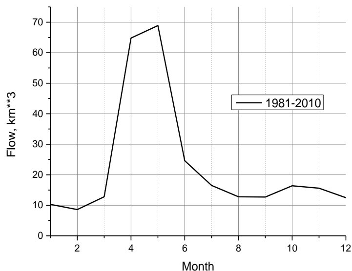
Рисунок 4. Многолетний сезонный ход стока Волги
