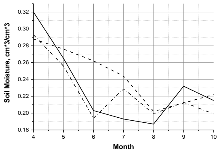
Рисунок 3. Сезонный ход средней влажности почв Волжского бассейна в 2015-2017 годах (сплошная кривая – данные 2016 г., штрих-пунктирная кривая – данные 2015 г. и пунктирная кривая – данные 2017 г.)
