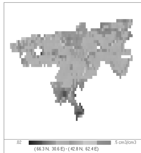
Рисунок 2. Распределения влажности почв Волжского бассейна по данным SMAP измерений
