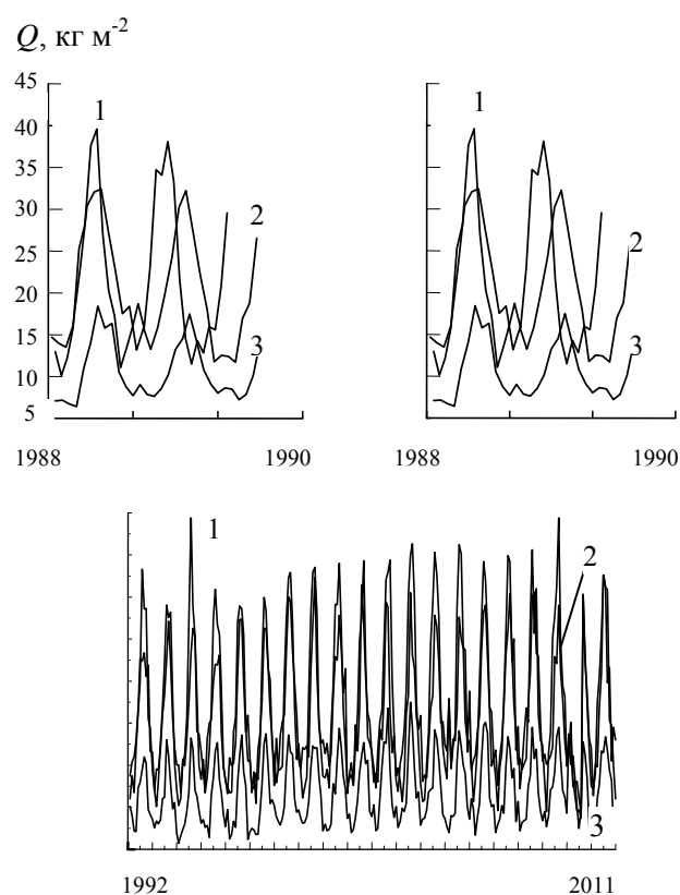
Рис. 2. Промежуточный этап исследований многолетних вариаций среднемесячных значений общего содержания водяного пара в атмосфере Q в зонах Н (1), D (2), М (3) Северной Атлантики на 22-летнем периоде спутниковых измерений
