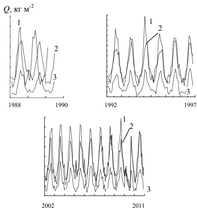
Рис. 1. Первоначальный этап исследований многолетних вариаций среднемесячных значений общего содержания водяного пара в атмосфере Q в зонах Н (1), D (2), М (3) Северной Атлантики на 22-летнем периоде спутниковых измерений
