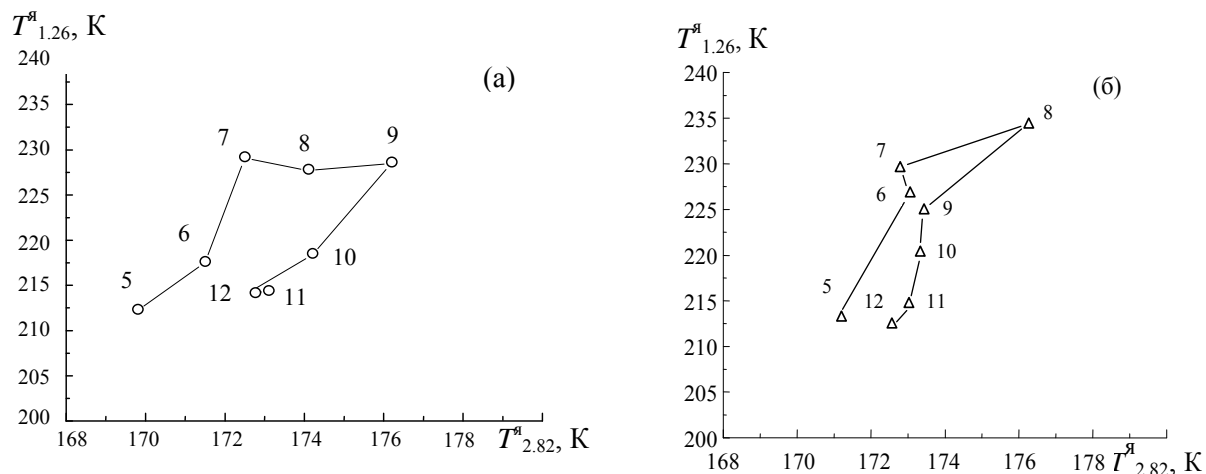
Рис. 4. Годовые траектории яркостной температуры на длинах волн 1,26 и 2,8 см в области D Северной Атлантики: (а) 2005 г.; (б) 2010 г. Цифры на рисунке – месяцы года
