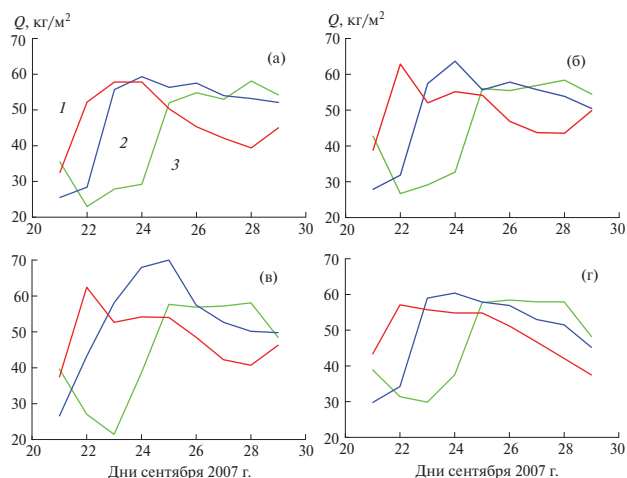
Рис. 1. Динамика ОВА ( Q ) в период, предшествующий зарождению ТУ Lorenzo в Мексиканском заливе в узлах сетки с координатами долготы 85.5^\circ з.д. (1), 91^\circ з.д. (2), 95.75^\circ з.д. (3) и широты 25^\circ с.ш. (а), 24^\circ с.ш. (б), 23^\circ с.ш. (в), 22^\circ с.ш. (г).
