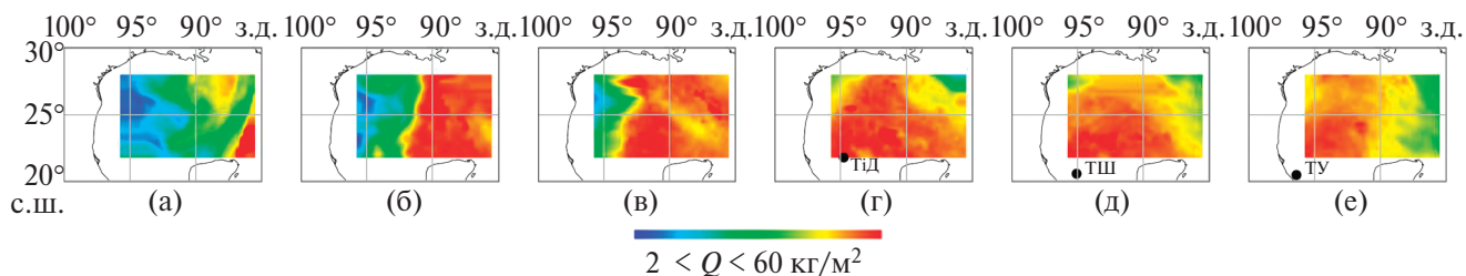
Рис. 2. Динамика изменения поля ОВА ( Q ) в выбранной области Мексиканского залива в период, предшествующий зарождению ТУ Lorenzo в сентябре 2007 г.: (а) – 22.09; (б) – 23.09; (в) – 24.09; (г) – 25.09; (д) – 26.09; (е) – 27.09. Время прихода тропической волны к Мексиканскому заливу 21 сентября. ТД – начало стадии тропической депрессии; ТШ – начало стадии тропического шторма; ТУ – начало стадии тропического урагана [Franklin, 2007].
