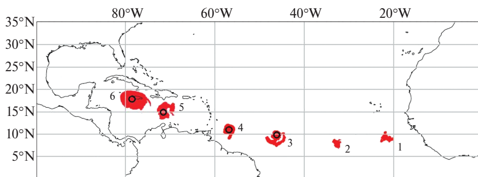
Рис. 5. Трансформация тропической волны в ТУ Ivan, 2004 г.: 1 – 01.09, 2 – 03.09, 3 – 05.09, 4 – 07.09, 5 – 09.09, 6 – 11.09. Выделенные области характеризуются ОВА 60 кг/м 2 и выше. Кружки отражают пространственное положение глаза урагана в полуденное время суток. По данным радиометра AMSR-E спутника EOS Aqua.
