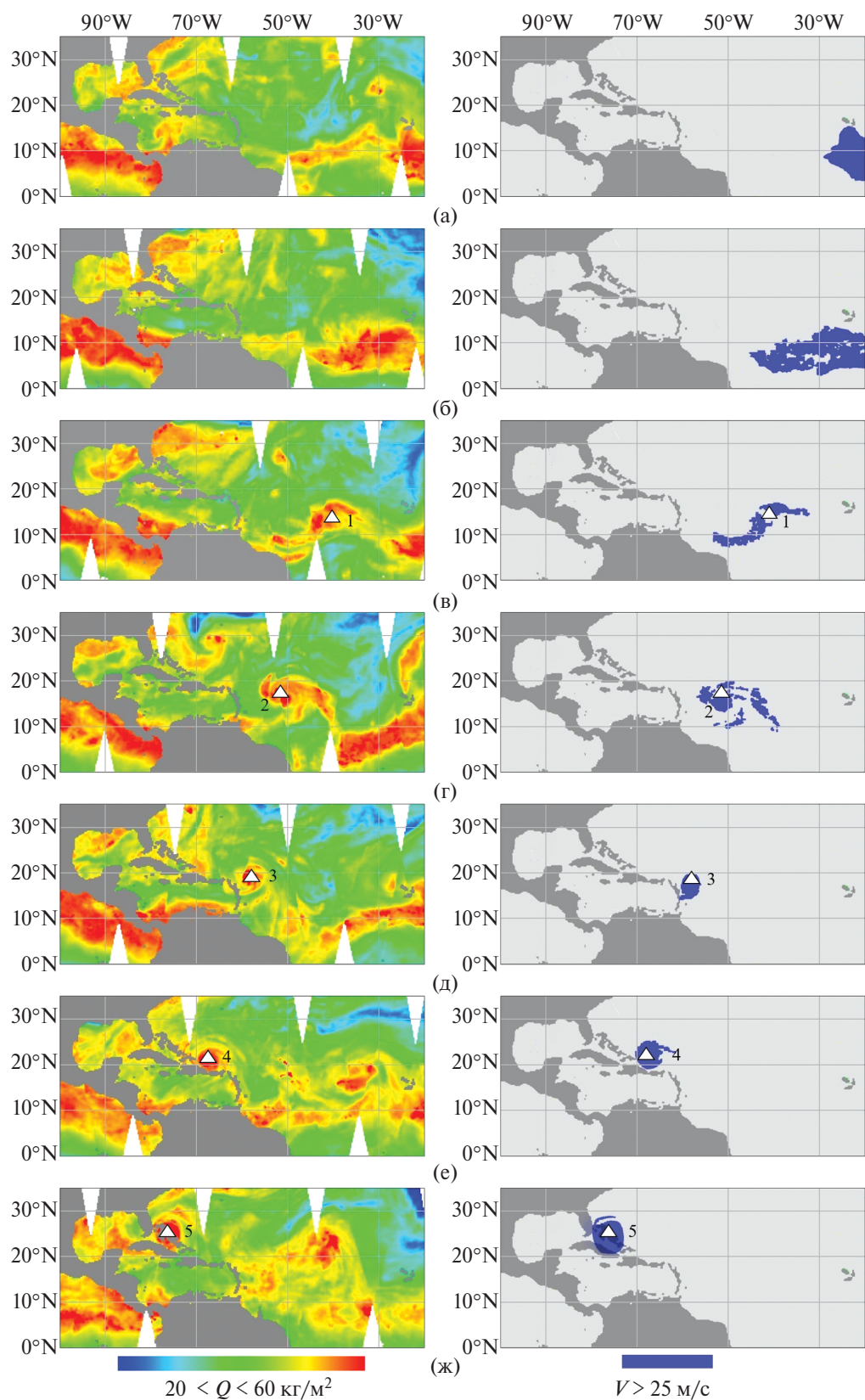
Рис. 7. Эволюция полей влажности атмосферы ( Q ) и скорости приводного ветра ( V ) в Атлантике по данным радиометра AMSR-E в период, предшествующий зарождению ТУ Frances: (а) – 22.08; (б) – 24.08 и его развития: (в) – 26.08; (г) – 28.09; (д) – 30.09; (е) – 01.09; (ж) – 03.09. 1 – тропический шторм; 2, 3, 4, 5 – тропический ураган (по данным [Beven II, 2014]). Белые клинообразные области – слепые зоны радиометра AMSR-E.
