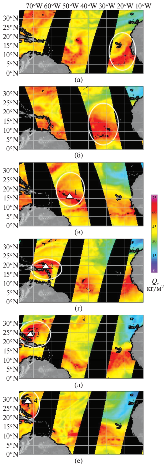
Рис. 6. Эволюции поля ОВА ( Q ) в тропической зоне Атлантики по данным измерений радиометров SSM/I спутников F11, F13, F14 на восходящих (A) и нисходящих (D) витках в период, предшествующий зарождению ТУ Bonnie: (а) – 15.08 (F14 D); (б) – 17.08 (F14 A); (в) – 19.08 (F11A); (г) – 21.08 (F13 D) и в период его развития: (д) – 23.08 (F14 D); (е) – 25.08 (F13D). 1 – тропическая депрессия; 2 – тропический шторм; 3, 4 – тропический ураган (по данным [Avila, 1998]). Слепые области (вне видимости радиометров) выделены черным цветом.
