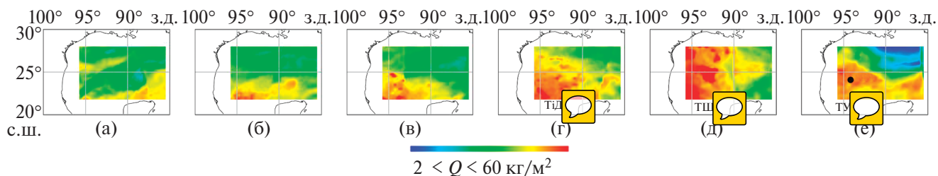
Рис. 3. Динамика поля ОВА ( Q ) в акватории Мексиканского залива в период, предшествующий зарождению тропического шторма Matthew в октябре 2004 г.: (а) – 03.10; (б) – 04.10; (в) – 05.10; (г) – 06.10; (д) – 07.10. Время прихода тропической волны к Мексиканскому заливу 3 октября. ТШ – начало стадии тропического шторма [Avila, 2004].
