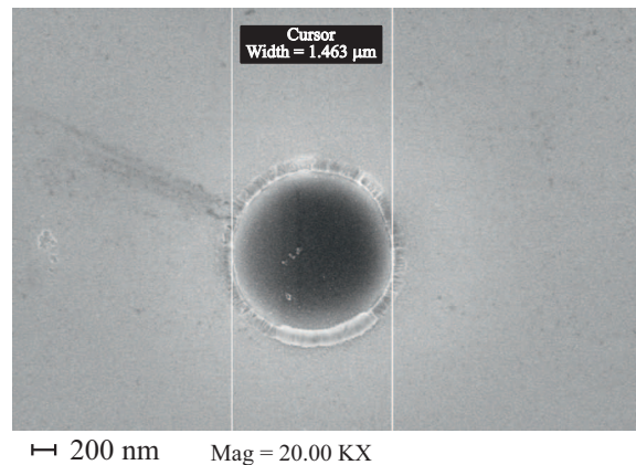
Рис. 2. Фотография СИС-перехода в СЭМ и измеренный диаметр перехода.
