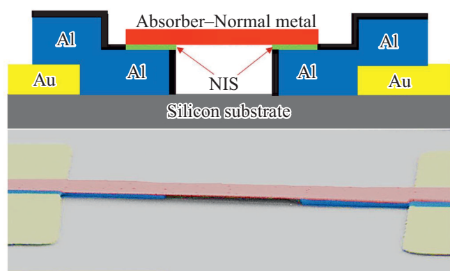
Рис. 2. Схематическое изображение болометра на основе СИНИС структуры и изображение изготовленной структуры в электронном микроскопе.
