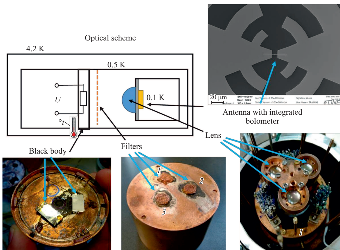
Рис. 4. Оптическая схема измерения отклика на внешнее излучение.
